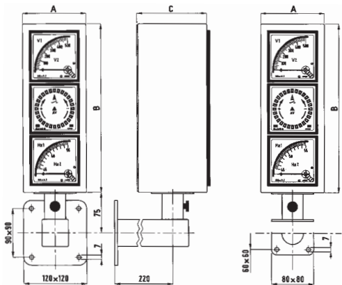
Dimensioni versione da incasso Flush mounting types - dimensions
